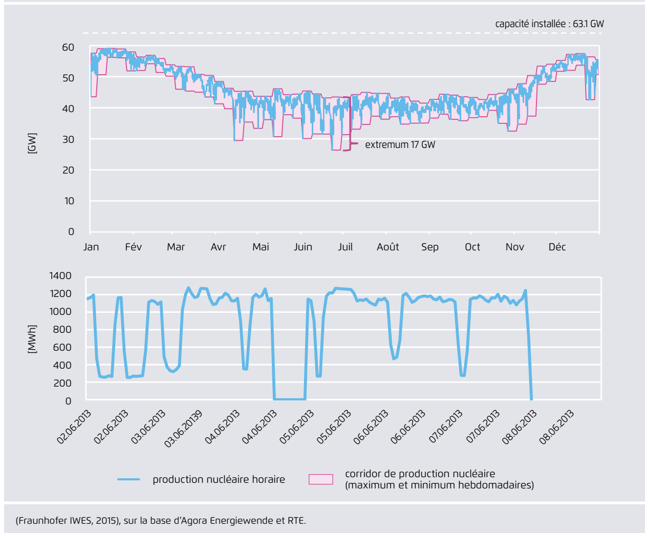
Variation annuelle de la production nucléaire en France en 2013 (haut) et exemple de la modulation de la puissance produite par un réacteur nucléaire sur une semaine en Juin 2013 (bas) Figure 5
