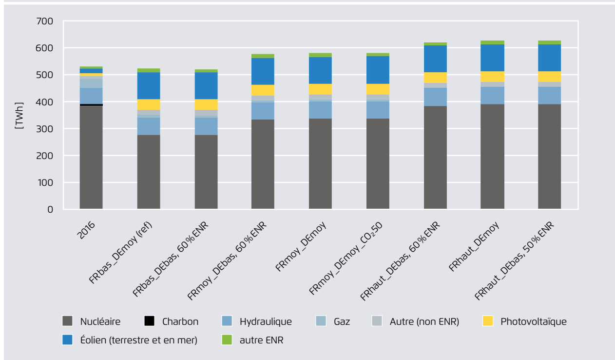
Production électrique en France en 2016 dans les différents scénarios 2030
