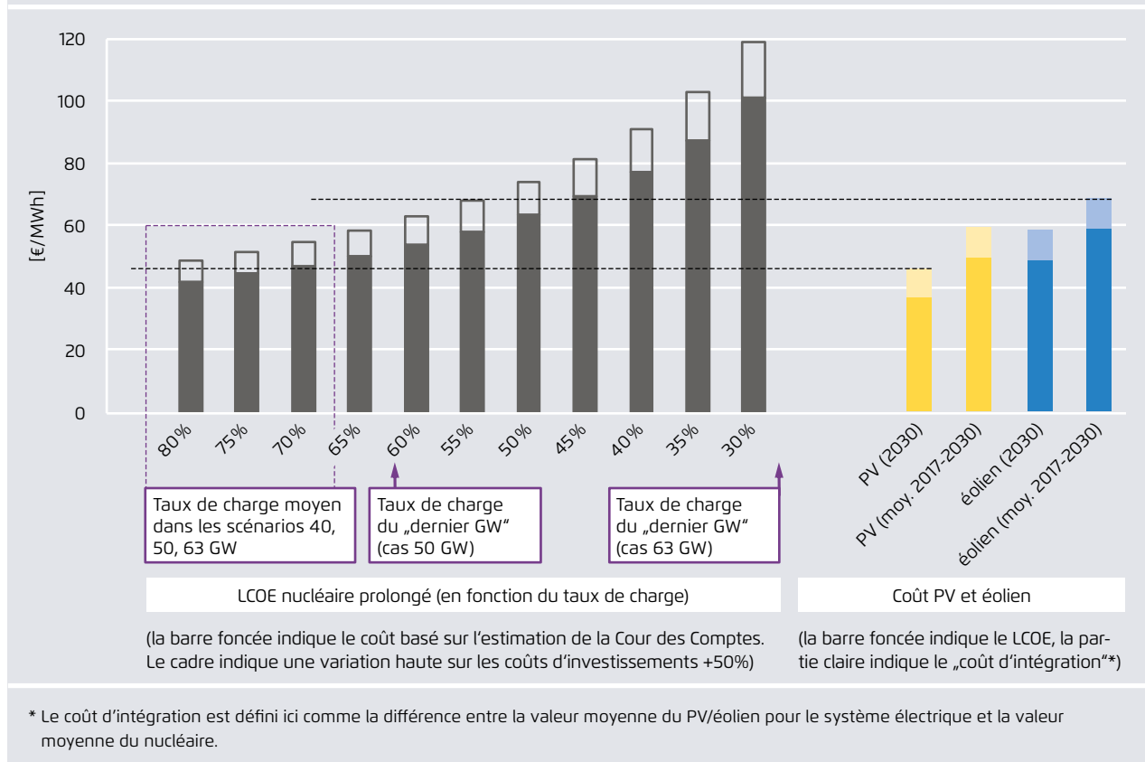
LCOE du nucléaire prolongé en fonction du taux de charge des réacteurs comparés aux alternatives photovoltaïque au sol et éolienne terrestre (avec prise en compte des « coûts d'intégration ») Figure 32
