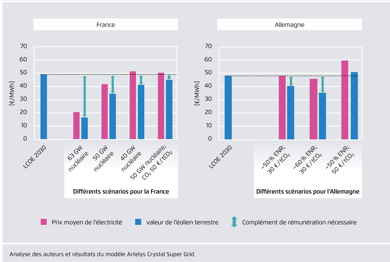
Prix de l'électricité et rémunération de l'éolien terrestre en 2030 en France (gauche) et en Allemagne (droite)
