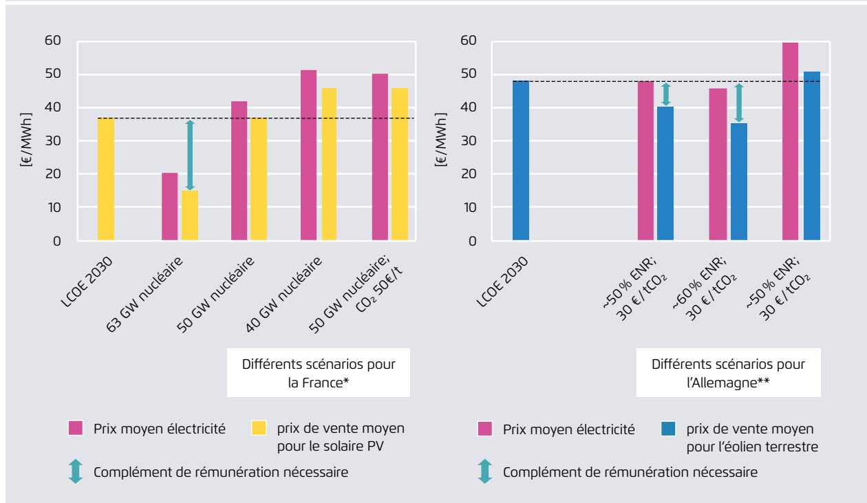
Prix de l'électricité et rémunération du PV en France en 2030 (gauche) et de l'éolien en Allemagne en 2030 (droite)
