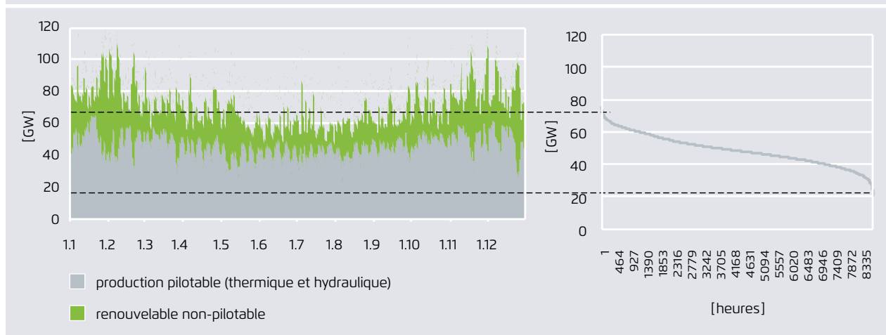
Production électrique annuelle en Allemagne en 2016 (gauche) et monotone de production résiduelle correspondante (droite)
