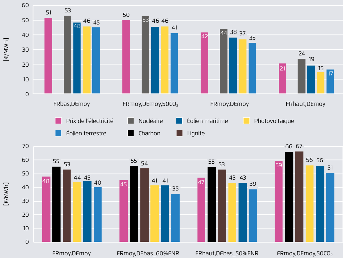
Rémunération de différentes filières de production dans les différents scénarios étudiés en France (haut) et en Allemagne (bas) en 2030
