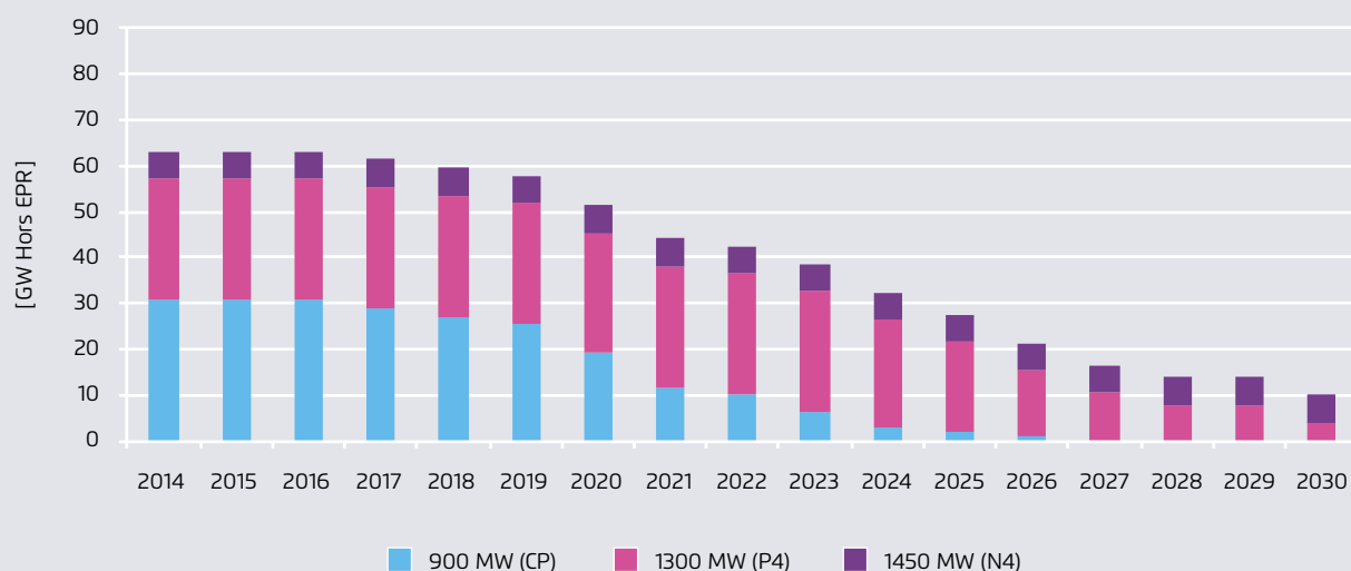
Évolution anticipée des capacités nucléaires existantes mises en service il y a moins de 40 ans si les réacteurs ne sont pas prolongés
