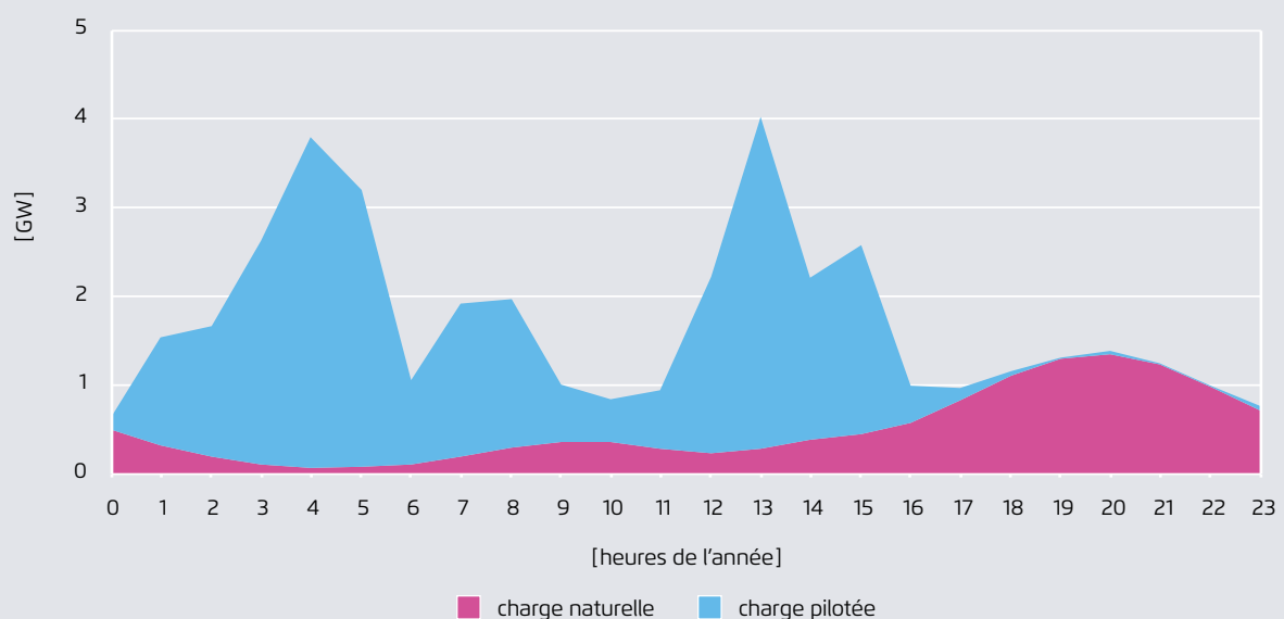
Profil de charge moyen des véhicules électriques en Allemagne (GW) en 2030 (scénario 50 % ENR) Figure A 5
