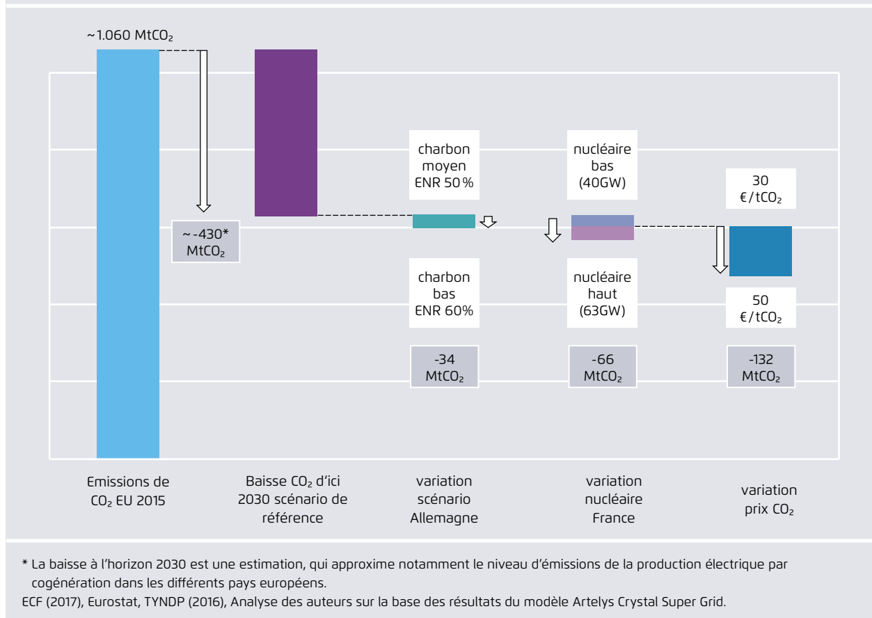
Baisse des émissions de CO 2 en Europe entre 2015 et 2030 dans différents scénarios étudiés
